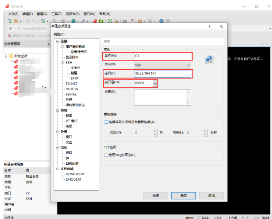
图 14 新建会话属性
