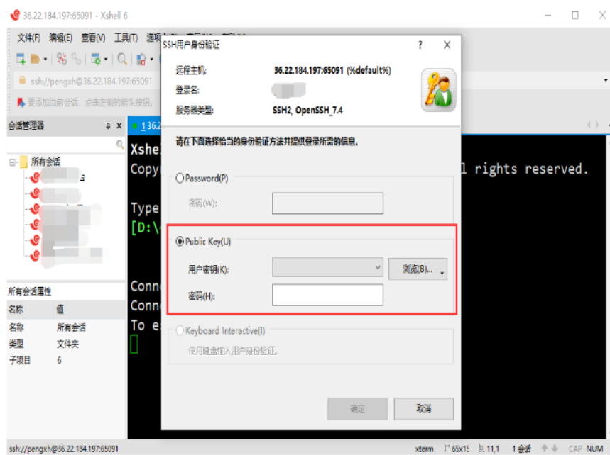
图 7 Public Key(U) 登录方式
