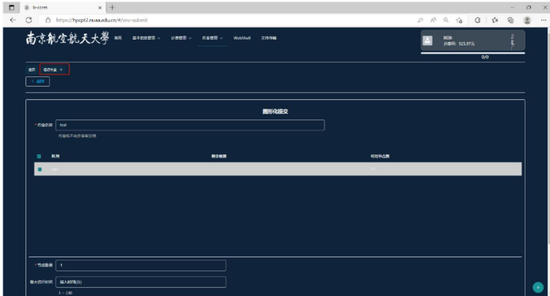
图 26 提交作业 3
