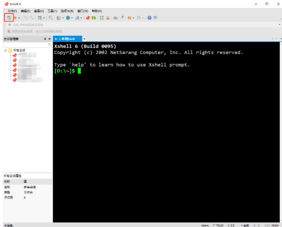
图 9 新建连接
