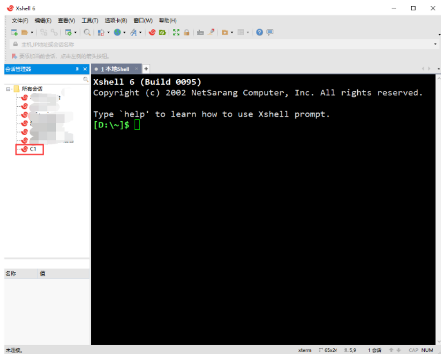
图 12 选择会话
