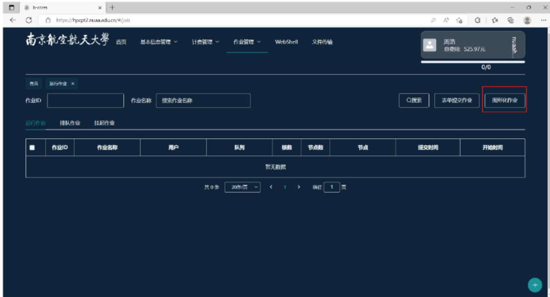
图 24 提交作业 1
