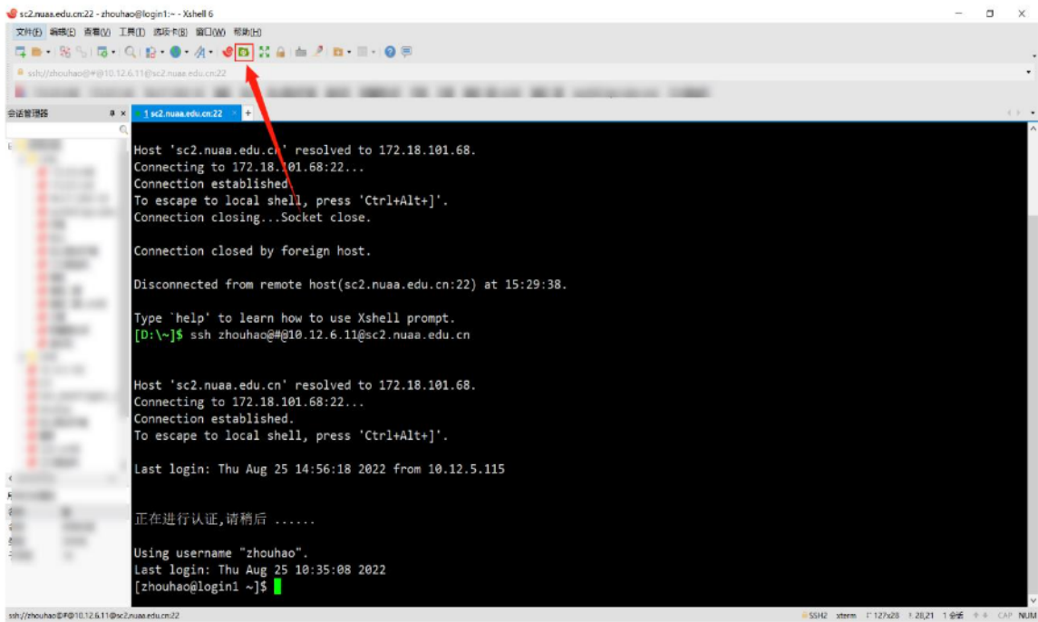
图 17 文件下载
