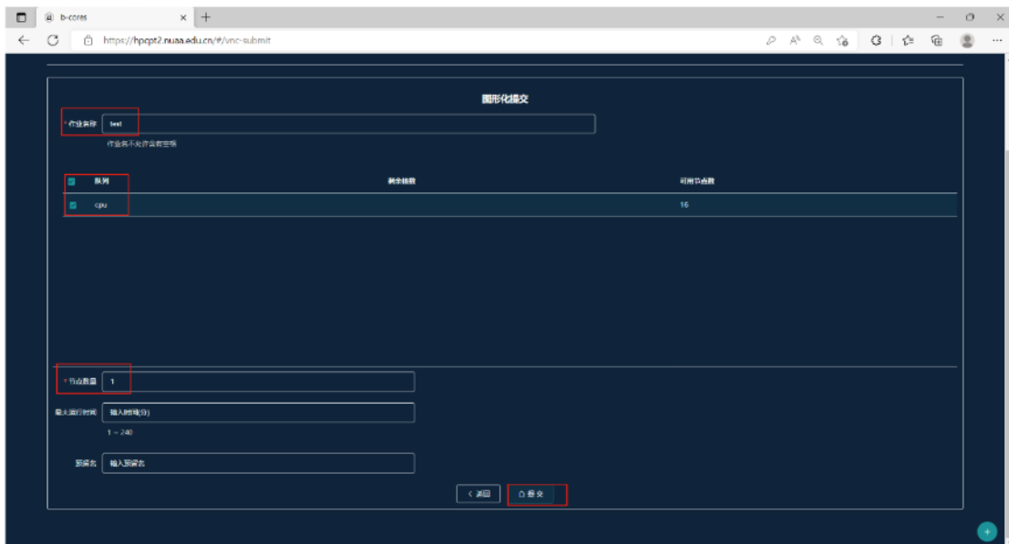
图 25 提交作业 2
