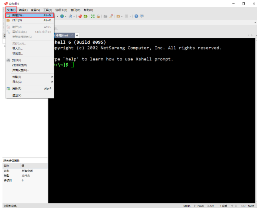
图 10 文件-连接
